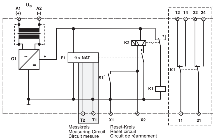
Fig. 1: Schematisches Schaltbild
