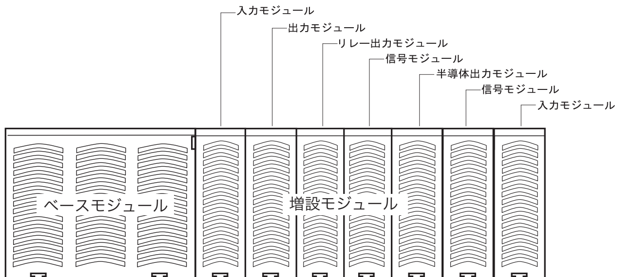
図 5-2: モジュラ式安全コントローラ PNOZmulti の例
