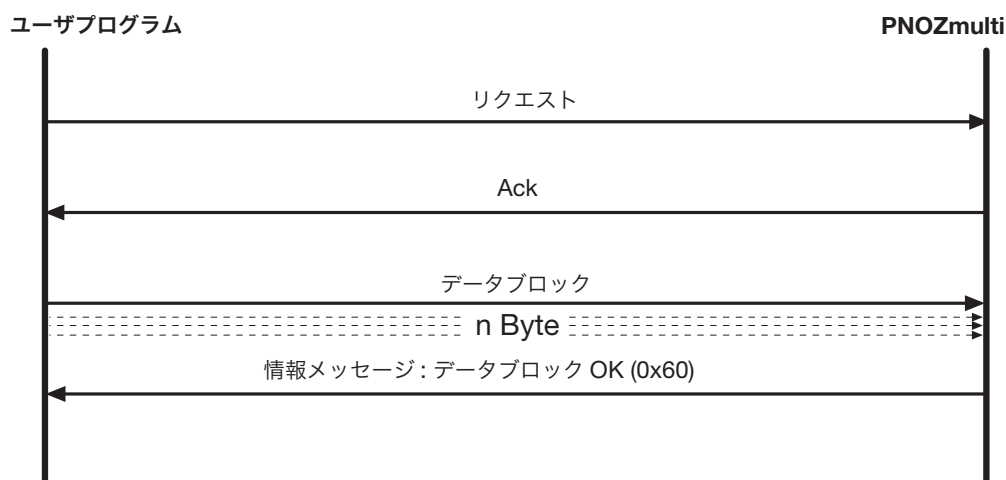
図 4-1: 通信の手順
