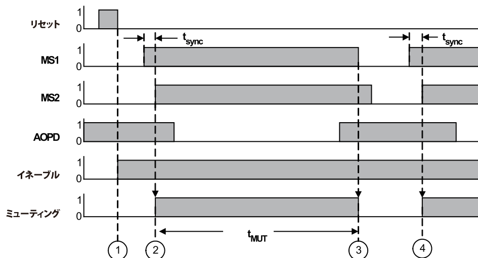
タイミングダイアグラム (例)
