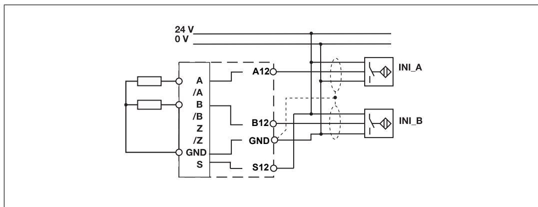
Capteurs de proximité pnp avec résistance R = 10\text{ k}\Omega
