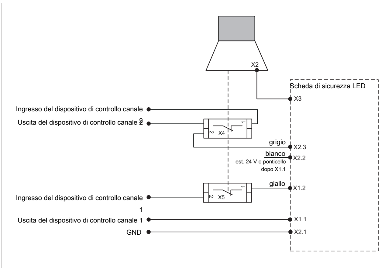
Fig.: Esempio di collegamento, la funzione di lampeggiamento non è attiva
