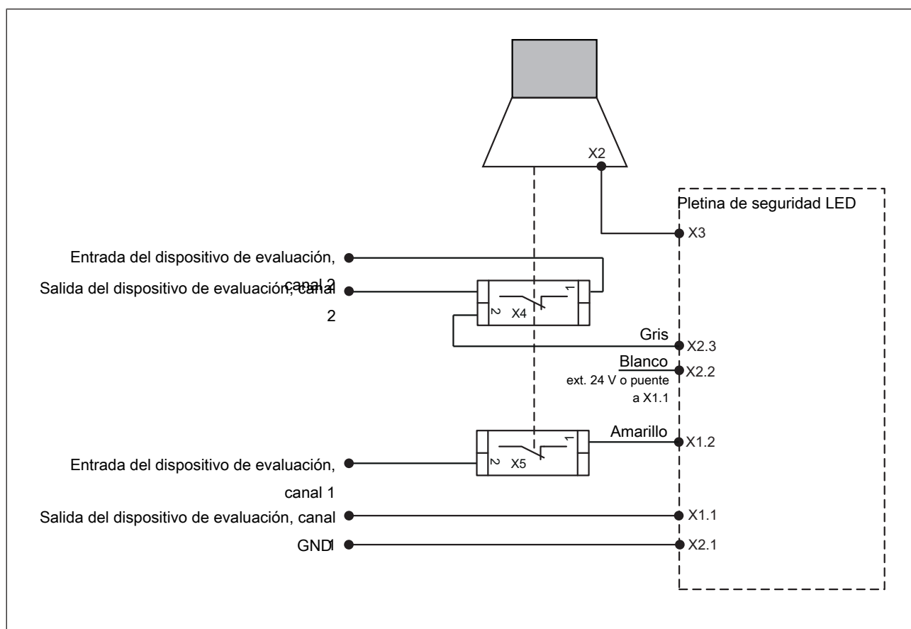
Fig.: Ejemplo de conexión, función de parpadeo inactiva
