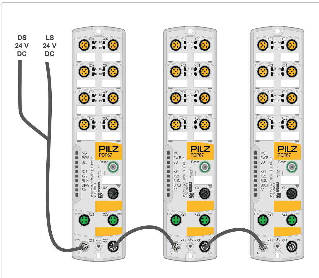
Fig.: Transmisión de la tensión de alimentación
