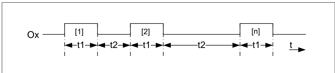
Fig.: Test asimétrico (se ejecuta solo en condiciones de funcionamiento sin fallos). El poder de corte de O+ y O- se comprueba mediante tests separados.
