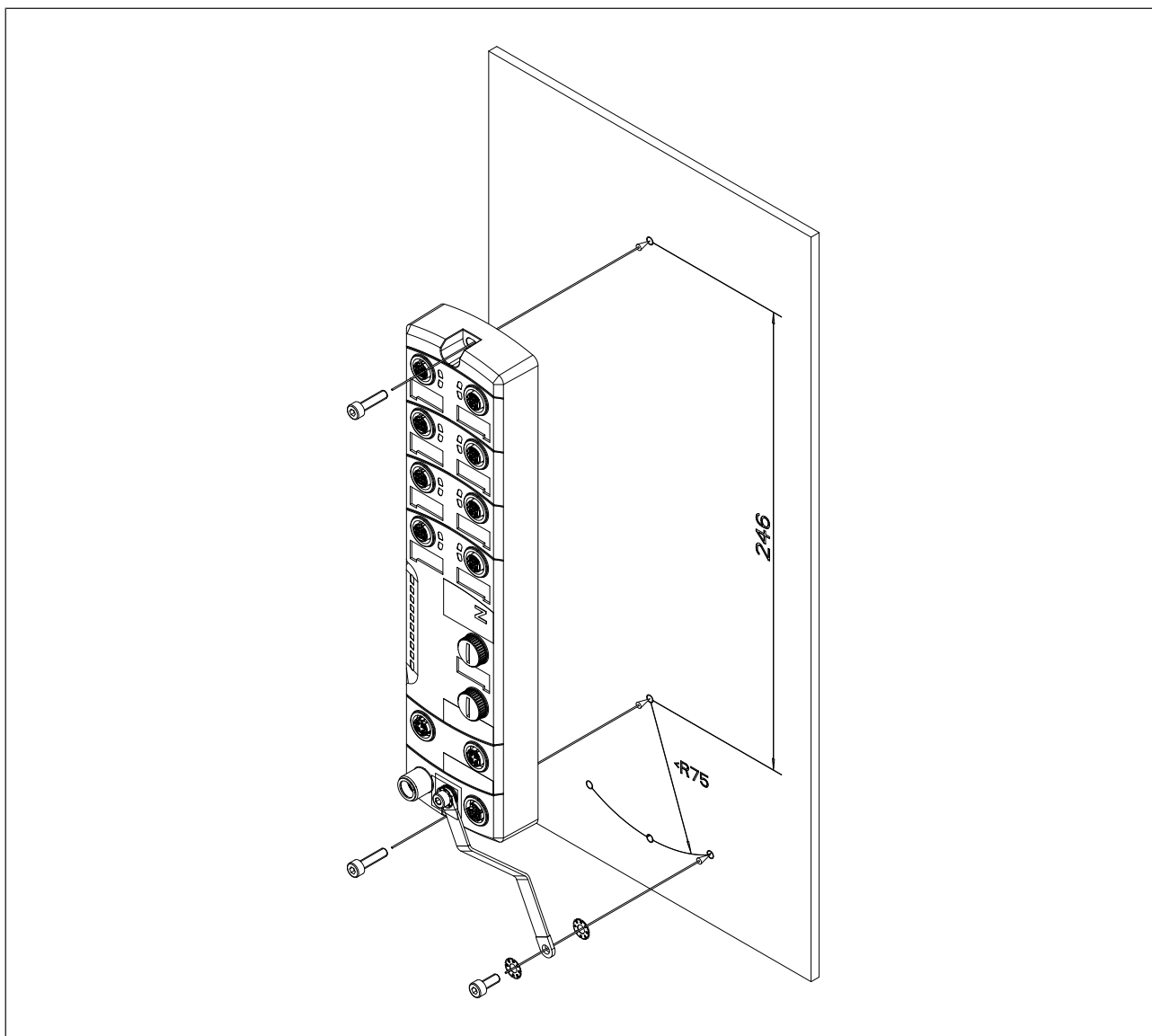
Fig.: Fijación en mm
