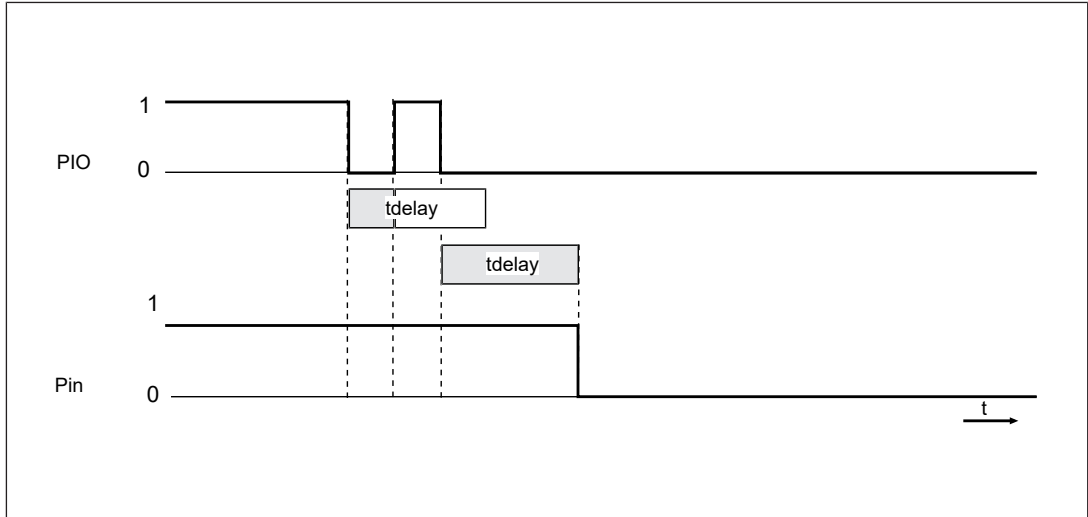
Fig.: Retardo a la desconexión
