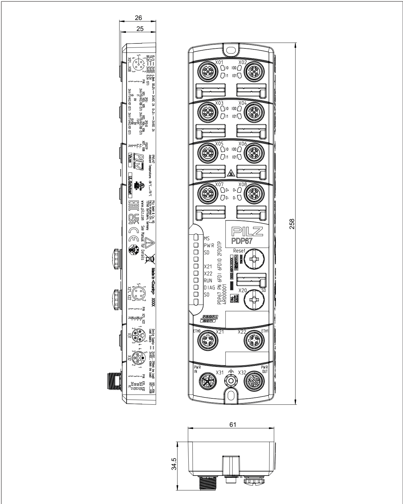
Fig.: Dimensions
