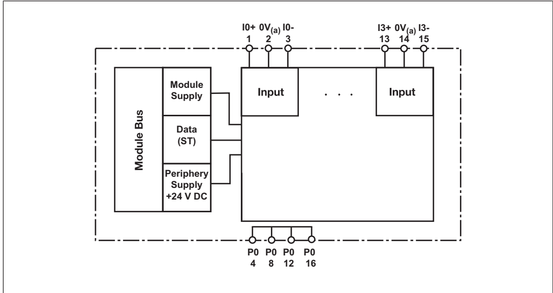
Fig.: Block diagram PSS u2 ES 4AI I (-R)
