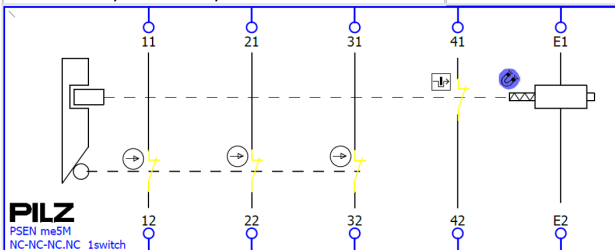
PSEN me5M NC-NC-NC-NC 1switch Bestell-Nr. / Order no. / Référence: 6L000011
