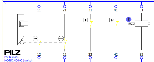
PSEN me5S NC-NC-NC-NC 1switch Bestell-Nr. / Order no. / Référence: 6L000018
