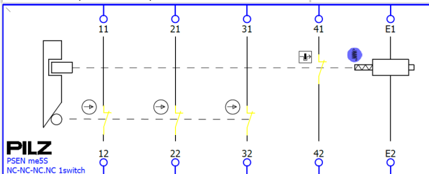
PSEN me5S NC-NC-NC-NC 1switch Bestell-Nr. / Order no. / Référence: 6L000010
