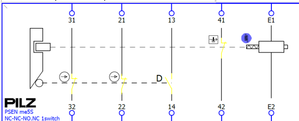
PSEN me5S NC-NC-NO-NC 1switch Bestell-Nr. / Order no. / Référence: 6L000014
