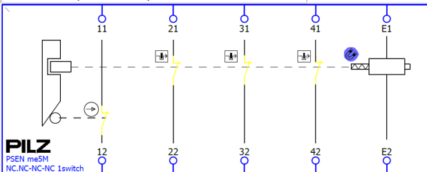
PSEN me5M NC-NC-NC-NC 1switch Bestell-Nr. / Order no. / Référence: 6L000013
