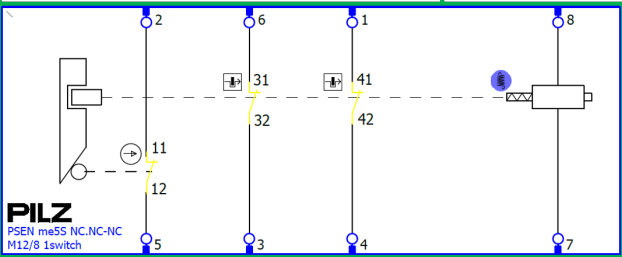
PSEN me5S NC.NC-NC M12/8 1switch Bestell-Nr. / Order no. / Référence: 6L000019
