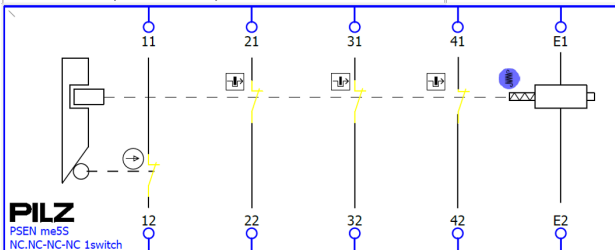
PSEN me5S NC-NC-NC-NC 1switch Bestell-Nr. / Order no. / Référence: 6L000012
