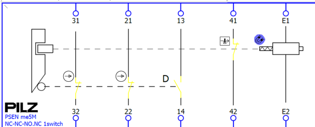
PSEN me5M NC-NC-NO-NC 1switch Bestell-Nr. / Order no. / Référence: 6L000015
