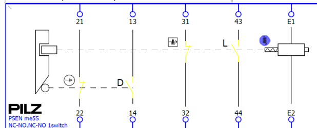
PSEN me5S NC-NO-NC-NO 1switch Bestell-Nr. / Order no. / Référence: 6L000016
