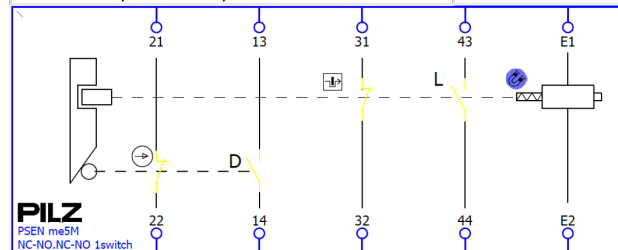
PSEN me5M NC-NO-NC-NO 1switch Bestell-Nr. / Order no. / Référence: 6L000017
