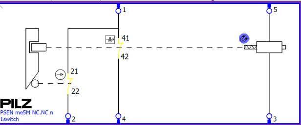
PSEN me5M NC.NC n 1switch Bestell-Nr. / Order no. / Référence: 6L000021
