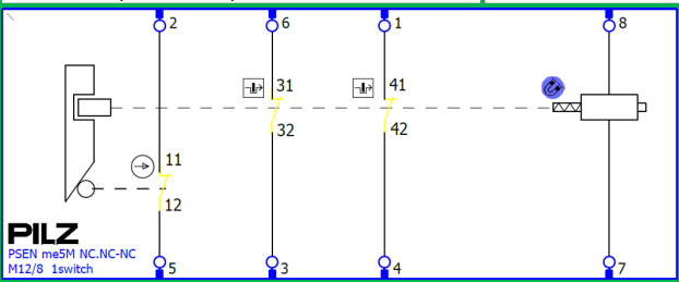
PSEN me5M NC.NC-NC M12/8 1switch Bestell-Nr. / Order no. / Référence: 6L000020
