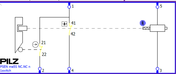
PSEN me5S NC.NC n 1switch Bestell-Nr. / Order no. / Référence: 6L000022
