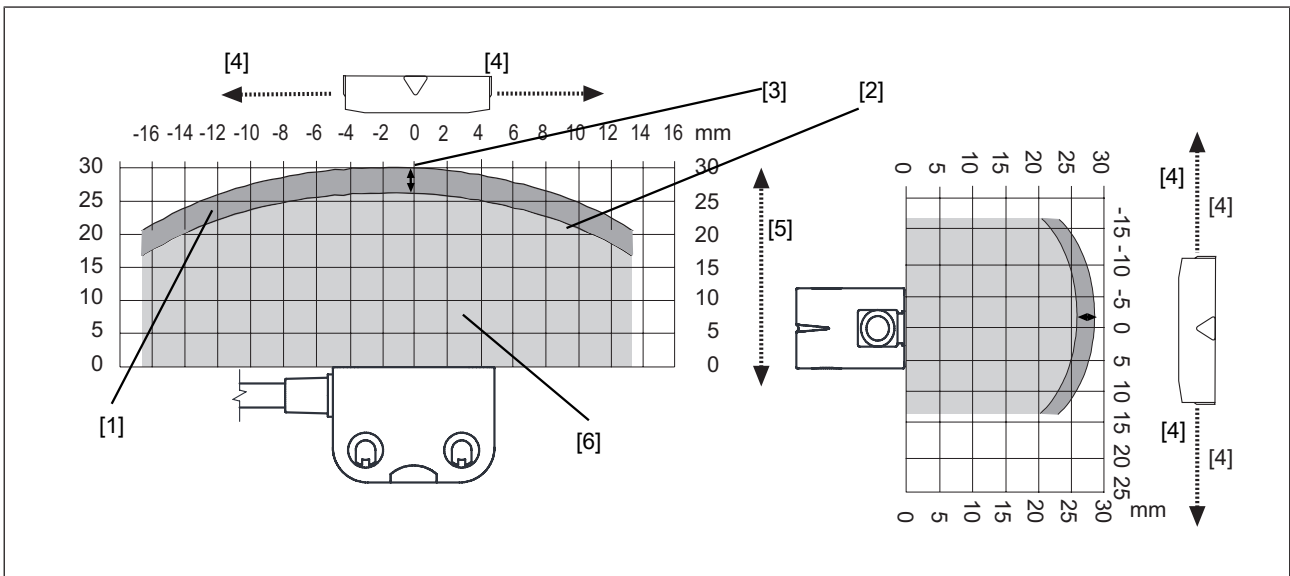
Illustration: Capteur de sécurité PSEN cs3.1a/b avec actionneur PSEN cs1.1
