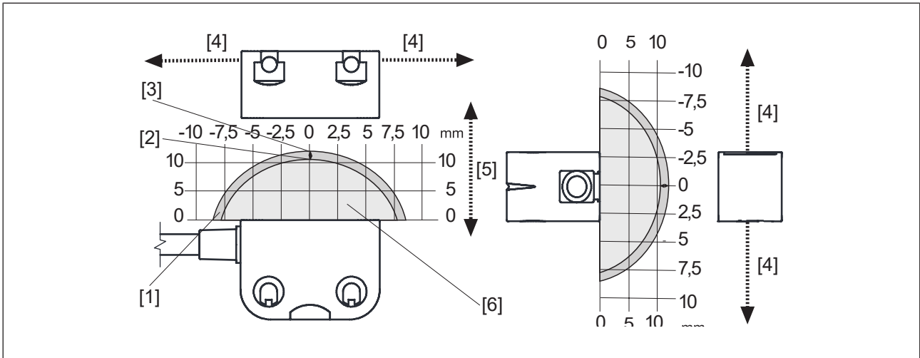
Illustration: Capteur de sécurité PSEN cs3.1a/b avec actionneur
